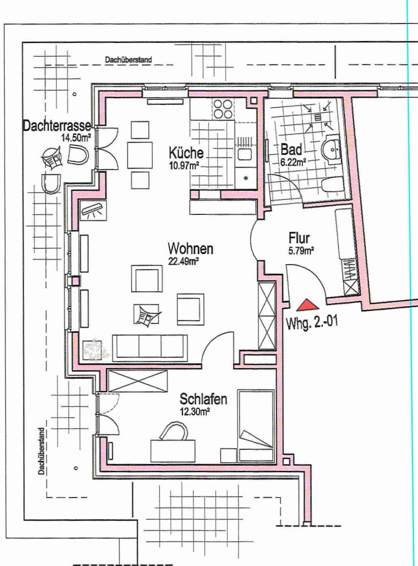
Staffelgeschoss Wohnung Nr. 2-01 M. 1:100 Wohnfläche 72.27 m 2
